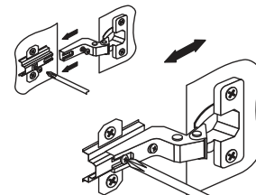
Регулировка створки по глубине
